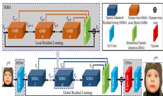
轻量级多尺度聚合图像超分辨率网络
