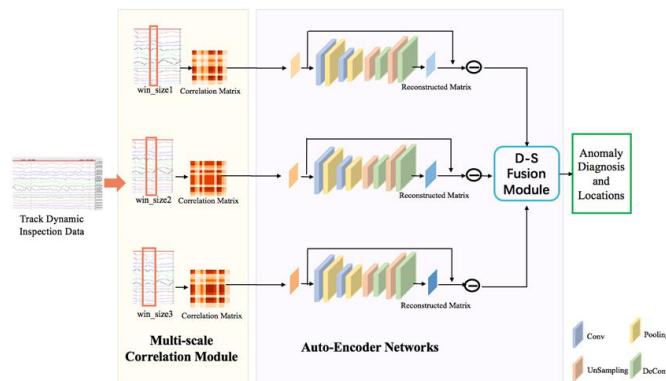
基于自动编码器和多尺度融合的轨检数据异常检测模型
