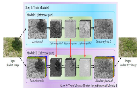
亮度引导去阴影模型LG-ShadowNet
