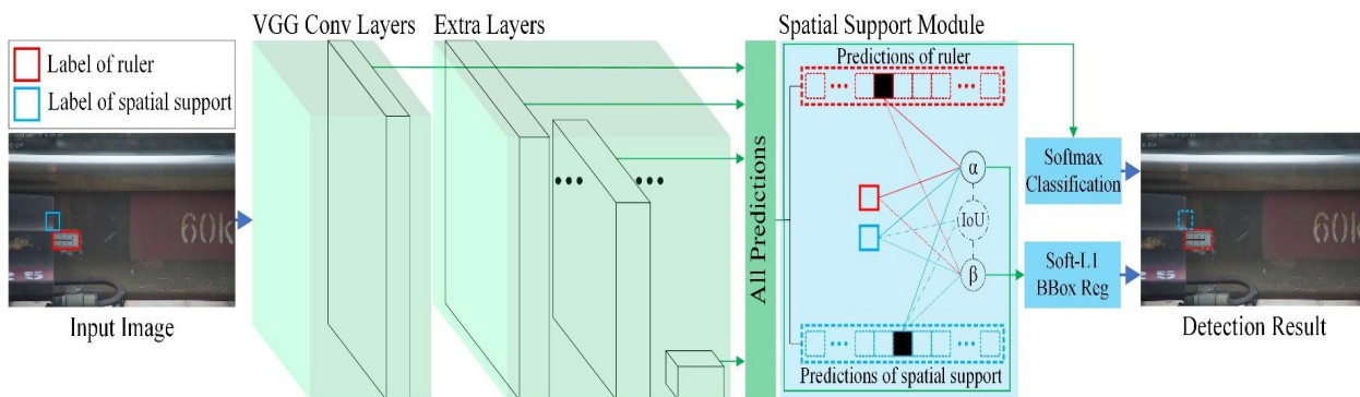
基于空间支撑的RCNN目标检测定位模型
