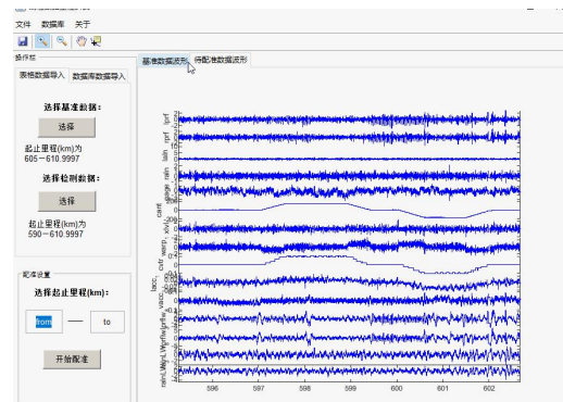
基于自动编码器和多尺度融合的轨检数据异常检测模型
