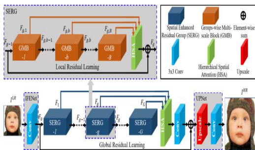
轻量级多尺度聚合图像超分辨率网络结构
